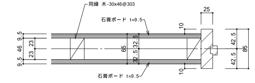
特記無き場合、これに準ずる 間仕切壁詳細 1/5
