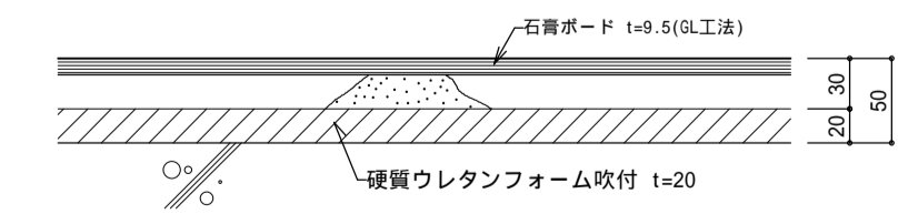
特記無き場合、これに準ずる 防露壁詳細 1/5
